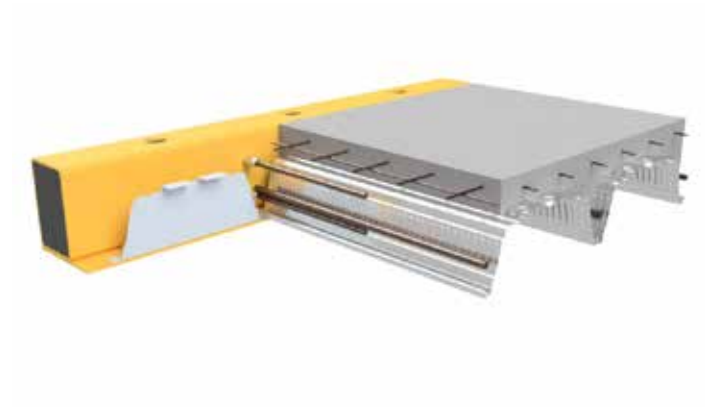
RHS edge beam SlimDek 210® perpendicular
